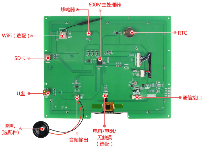
图 1-4 硬件配置图
