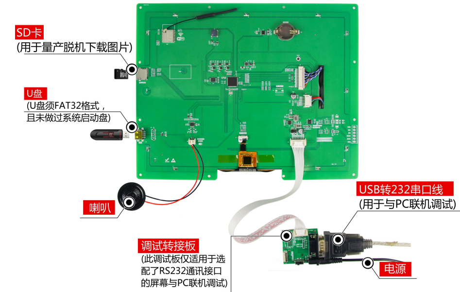
图 1-5 调试工具图
